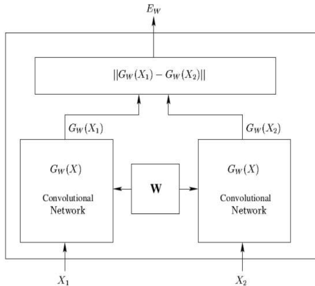
Hình 1.11: Mô hình tiếp cận Deep learning cho học độ đo khoảng cách
