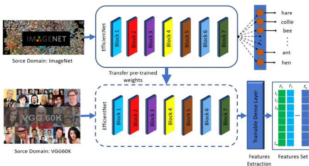
Hình 1.6: Mô hình trích rút đặc trưng ảnh bằng mô hình học sâu
