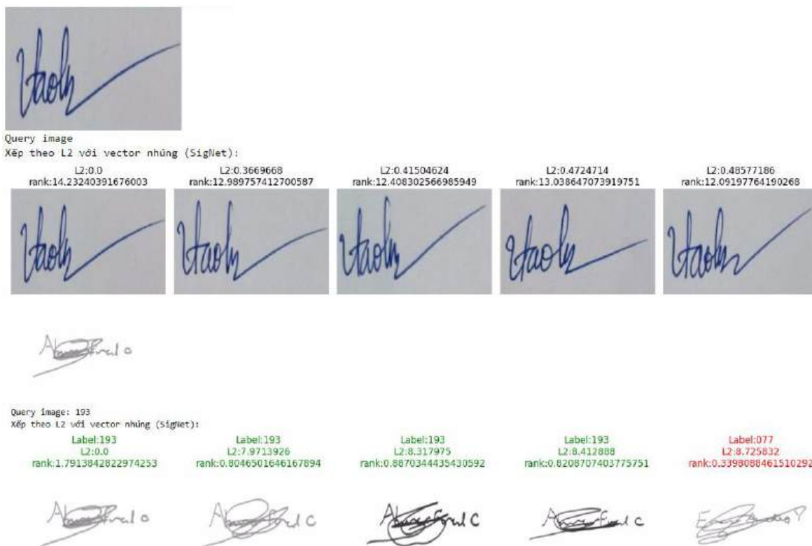
Hình 3.4: Kết quả so sánh độ tương tự ảnh chữ ký trong bộ Sign300HD sử dụng EMR Learning
