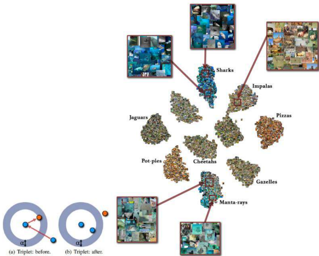
Hình 1.13 Chiến thuật Triplet phân loại ảnh
