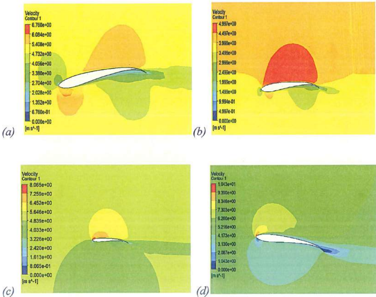
Hình 3.37. Đường đồng mức dòng khí và các dòng xoáy khí tương tác với bề mặt mẫu cánh VAST-EPU-S1010 với các góc: AoA = -5^\circ (a), AoA = -0^\circ (b), AoA = 5^\circ (c), AoA = 10^\circ (d) ở tốc độ gió 5,0 m/s
