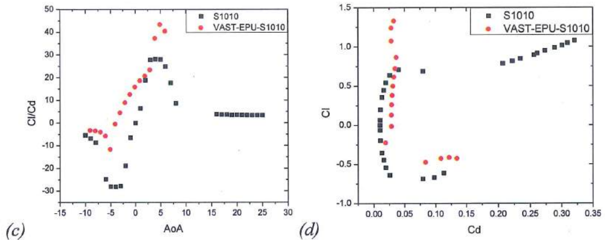
Hình 3.26. Các giá trị thu được của C_l (a), C_d (b), C_l/C_d (c), C_l so với C_d (d) của S1010 và VAST-EPU-S1010 khi hoạt động ở tốc độ gió 5,0 m/s
