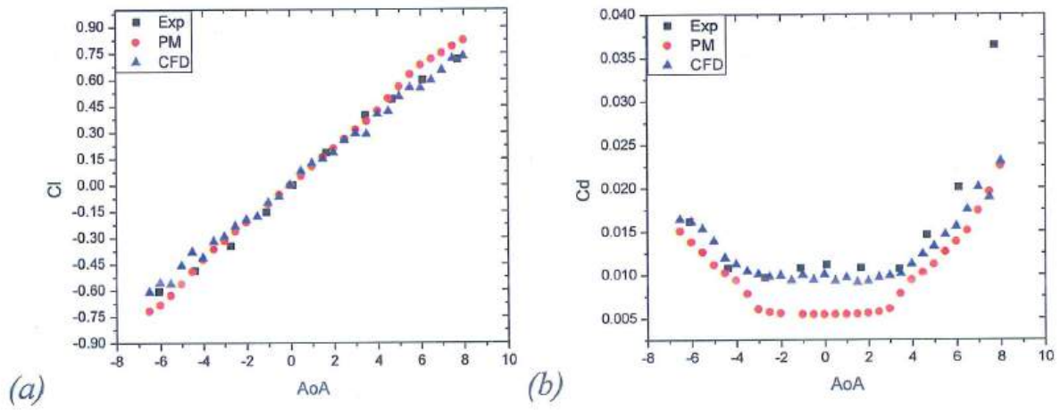
Hình 3.18. So sánh các thông số khí động học của NACA64A010 khi tốc độ gió là 4,78 m/s: C_l (a); C_d (b); C_l/C_d (c)
