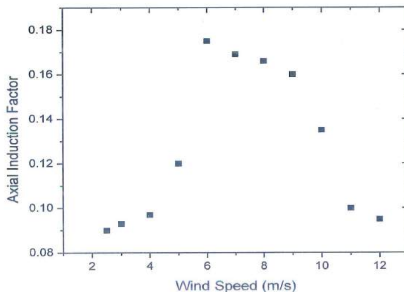
Hình 4.17. Hệ số cảm ứng hướng trục của E103 theo tốc độ gió
