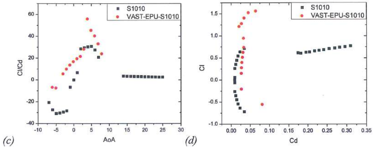
Hình 3.27. Các giá trị thu được của C_l (a), C_d (b), C_l/C_d (c), C_l so với C_d (d) của S1010 và VAST-EPU-S1010 khi hoạt động ở tốc độ gió 6,0 m/s
