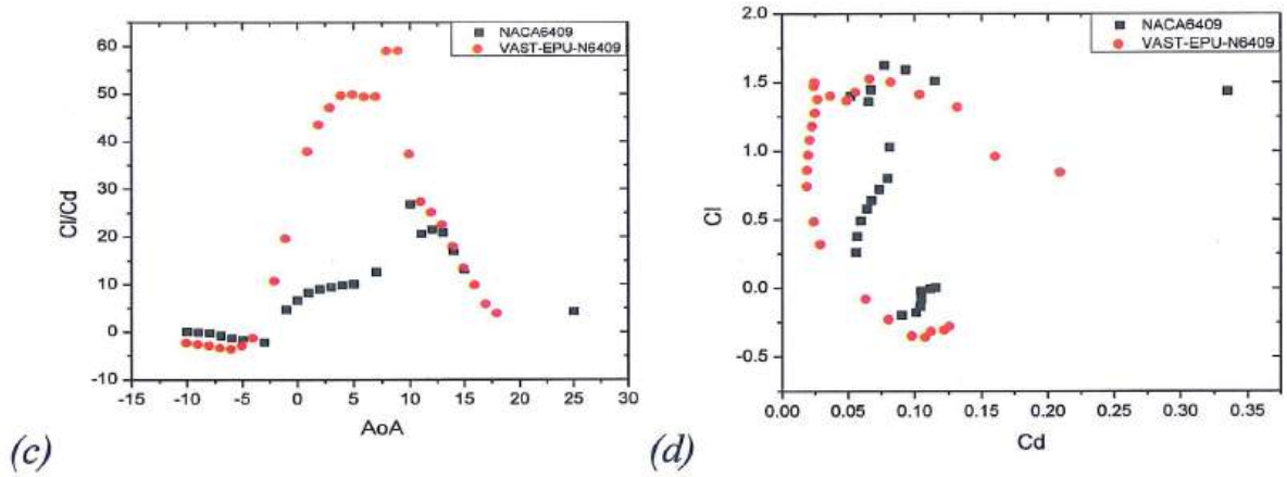
Hình 3.21. Các giá trị thu được của C_l (a), C_d (b), C_l/C_d (c), C_l so với C_d (d) của NACA6409 và VAST-EPU-N6409 khi hoạt động ở tốc độ gió 4,0 m/s
