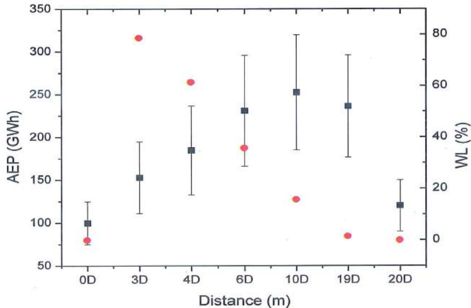
Hình 4.19. Thay đổi của AEP và WL theo các cấu hình lắp đặt khác nhau
