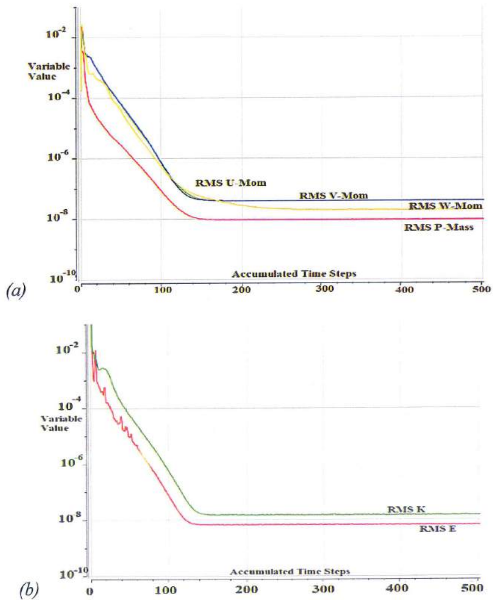
Hình 4.7. Thặng giá sai số của các đại lượng: tốc độ và động lượng (a); và k và \varepsilon (b)
