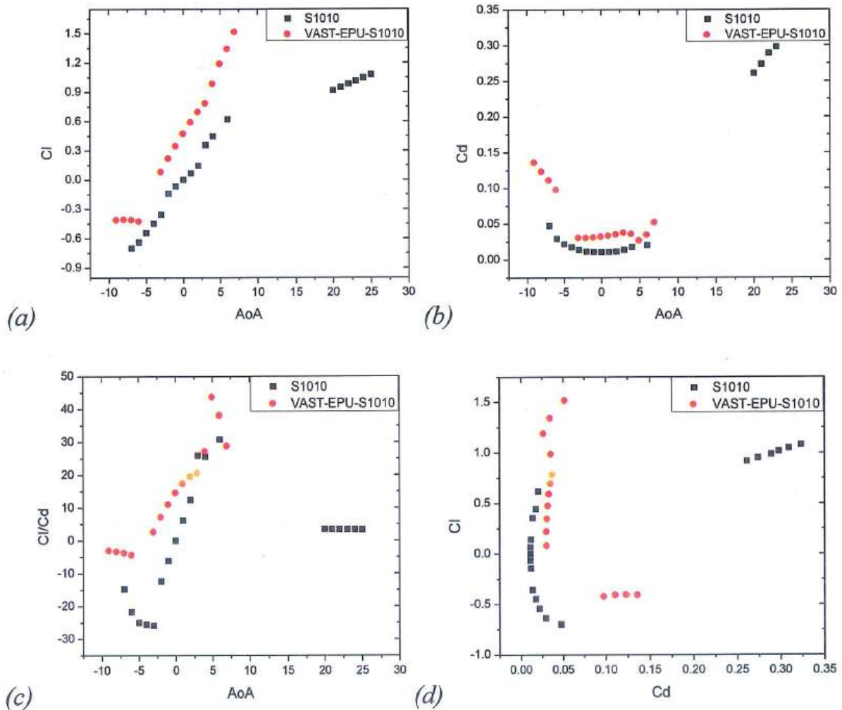
Hình 3.25. Các giá trị thu được của C_l (a), C_d (b), C_l/C_d (c), C_l so với C_d (d) của S1010 và VAST-EPU- S1010 khi hoạt động ở tốc độ gió 4,0 m/s
