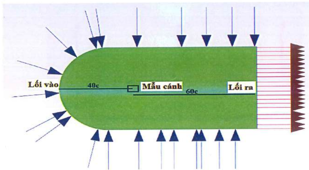
Hình 3.16. Mô hình mô phỏng CFD cho mẫu cánh
