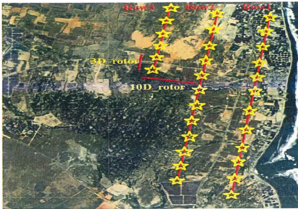
Hình 4.20. Cấu hình lắp đặt các tuabin E103 tối ưu tại trang trại
