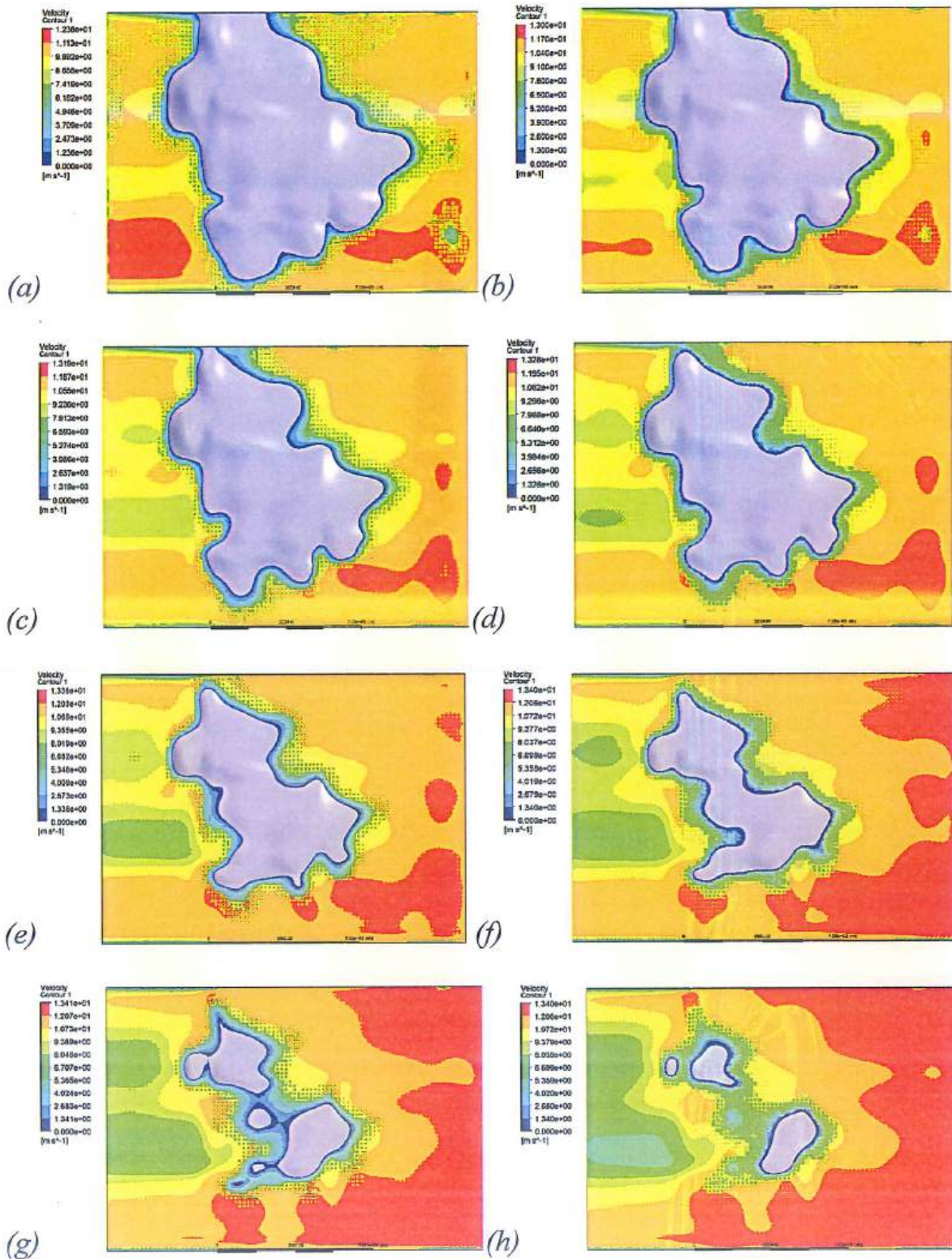
Hình 3.9. Phân bố tốc độ gió ở các độ cao khác nhau: (a) h=166 \text{ m} , (b) h=216 \text{ m} , (c) h=266 \text{ m} , (d) h=316 \text{ m} , (e) h=366 \text{ m} , (f) h=416 \text{ m} , (g) h=466 \text{ m} và (h) h=516 \text{ m}
