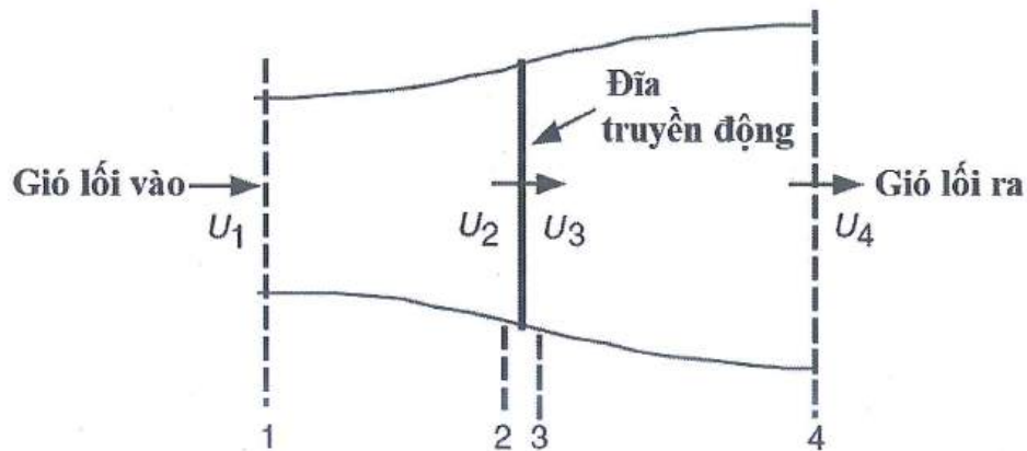
Hình 2.1. Mô hình minh họa lý thuyết BEM [48].
