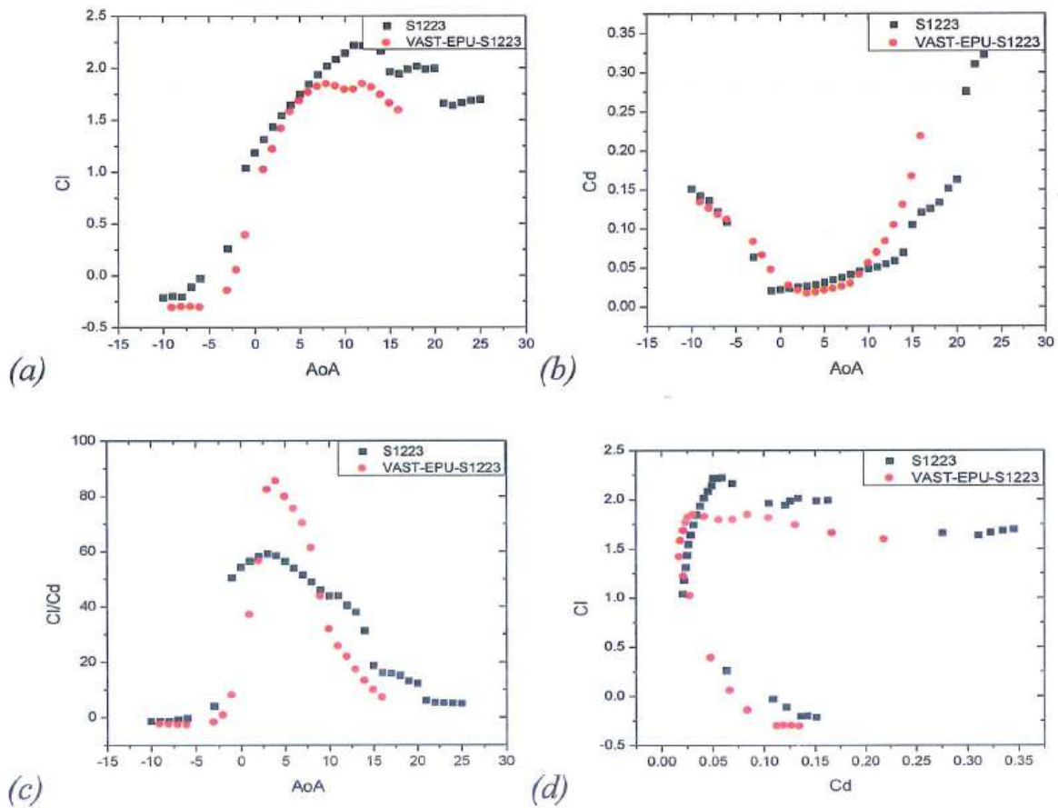
Hình 3.30. Các giá trị thu được của C_l (a), C_d (b), C_l/C_d (c), C_l so với C_d (d) của S1223 và VAST-EPU-S1223 khi hoạt động ở tốc độ gió 5,0 m/s
