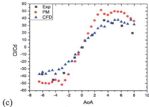
(c) Hình 3.19. So sánh các thông số khí động học của NACA64A010 khi tốc độ gió là 9,73 m/s: C_l (a); C_d (b); C_l/C_d (c)
