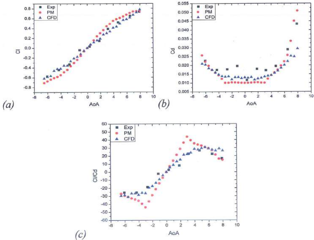
Hình 3.17. So sánh các thông số khí động học của NACA64A010 khi tốc độ gió là 2,96 m/s: C_l (a); C_d (b); C_l/C_d (c)
