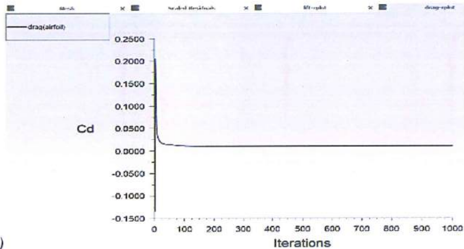
Hình 3.32. Sự thay đổi của các đại lượng theo số lần lặp: Sai số (a), hệ số lực nâng (b) và hệ số lực cản (c) theo các vòng lặp giải số
