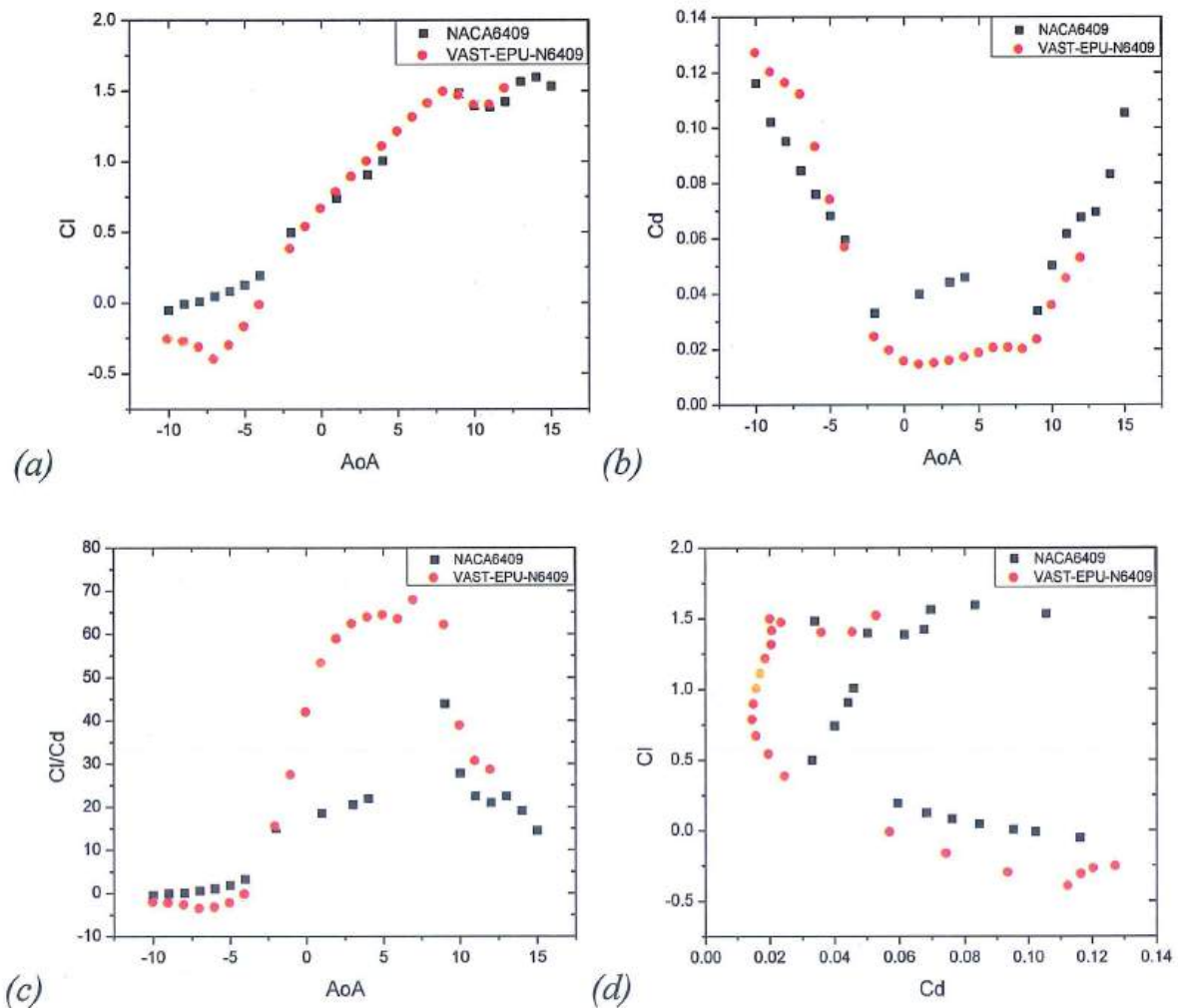
Hình 3.23. Các giá trị thu được của C_l (a), C_d (b), C_l/C_d (c), C_l so với C_d (d) của NACA6409 và VAST-EPU-N6409 khi hoạt động ở tốc độ gió 6,0 m/s
