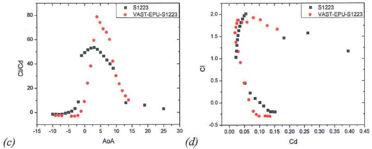
Hình 3.29. Các giá trị thu được của C_l (a), C_d (b), C_l/C_d (c), C_l so với C_d (d) của S1223 và VAST-EPU-S1223 khi hoạt động ở tốc độ gió 4,0 m/s
