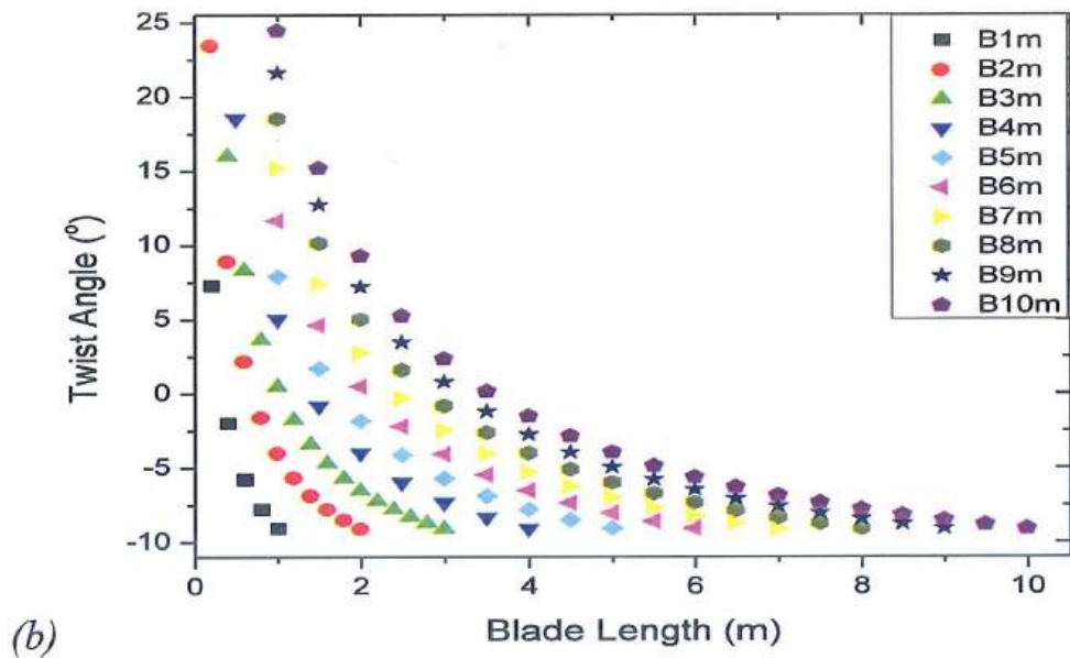
Hình 3.39. Mối liên hệ giữa chiều dài (a), góc xoắn (b) của các phần mẫu cánh SG6043 và chiều dài toàn bộ cánh quạt
