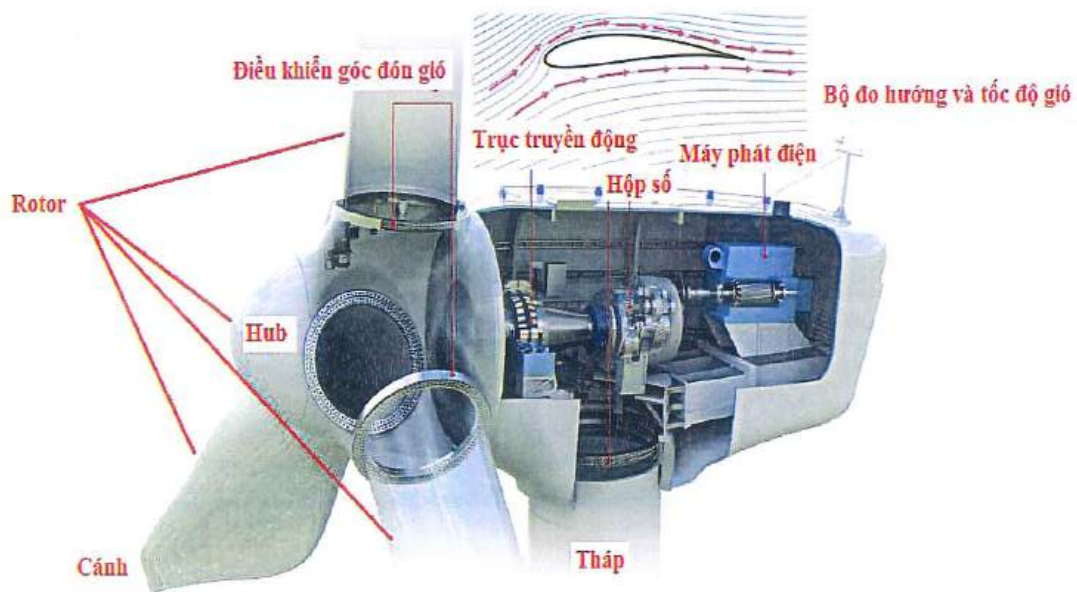
Hình 3.11. Minh họa các thành phần chính của tuabin trục ngang [72]
