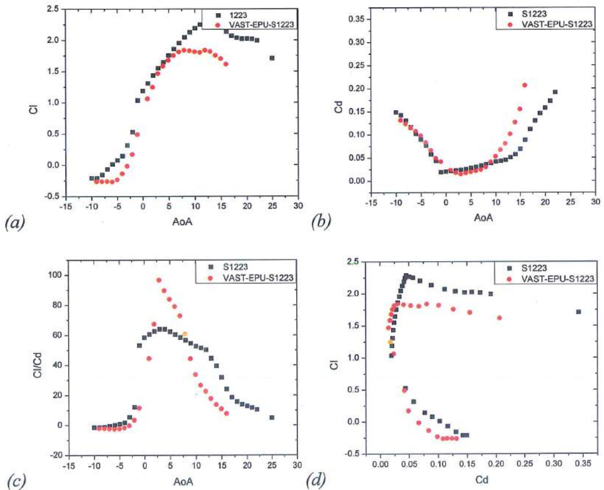
Hình 3.31. Các giá trị thu được của C_l (a), C_d (b), C_l/C_d (c), C_l so với C_d (d) của S1223 và VAST-EPU-S1223 khi hoạt động ở tốc độ gió 6,0 m/s
