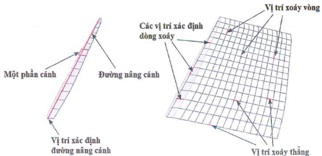
Hình 2.5. Minh họa phương pháp LLFVWM đối với cánh tuabin [56]
