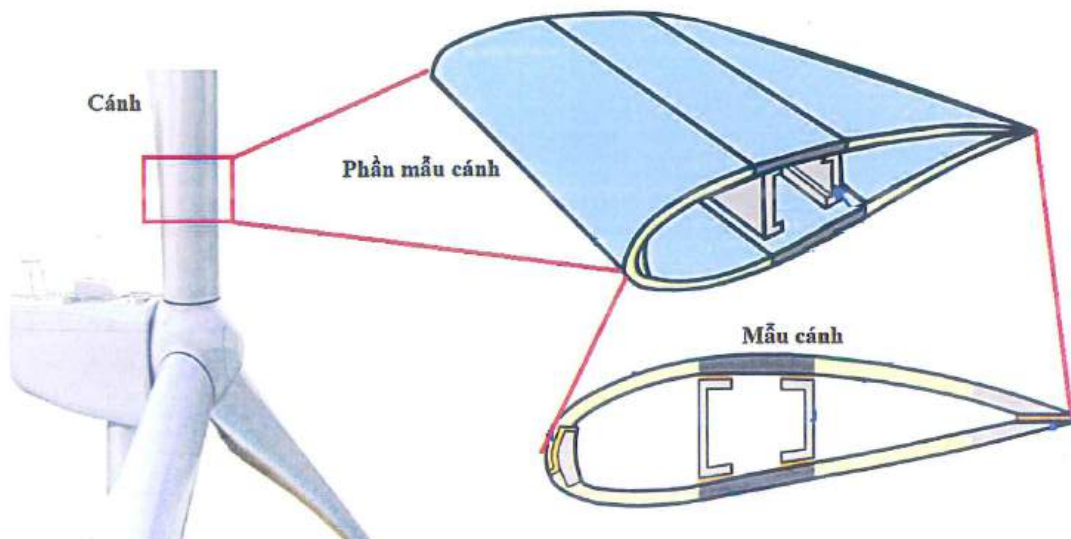
Hình 3.13. Minh họa thiết kế của một cánh tuabin gió trục ngang [73]
