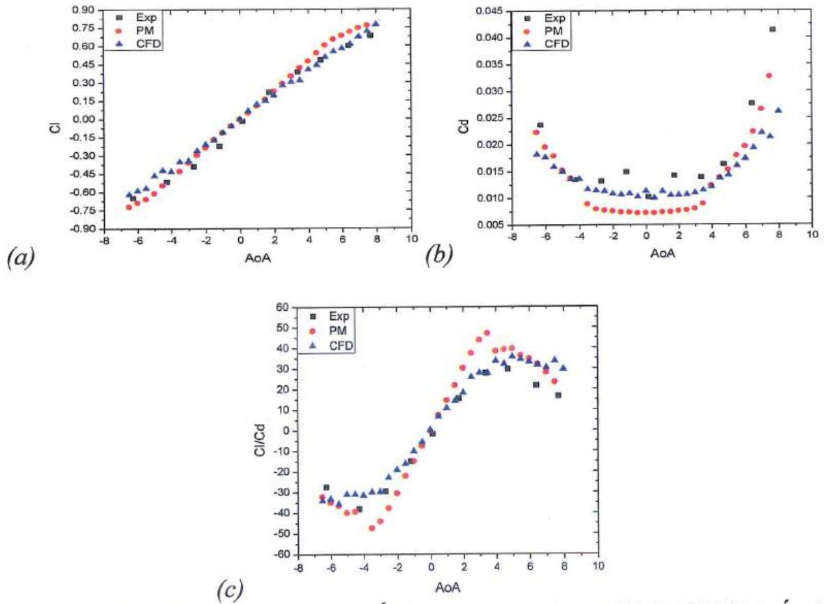
Hình 3.18. So sánh các thông số khí động học của NACA64A010 khi tốc độ gió là 4,78 m/s: C_l (a); C_d (b); C_l/C_d (c)
