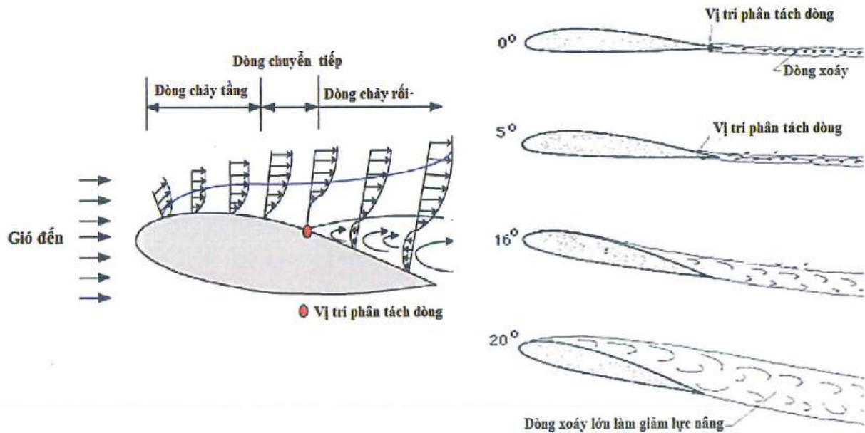
Hình 3.14. Minh họa quá trình tương tác giữa dòng chảy tới và phần mẫu cánh tuabin [48]
