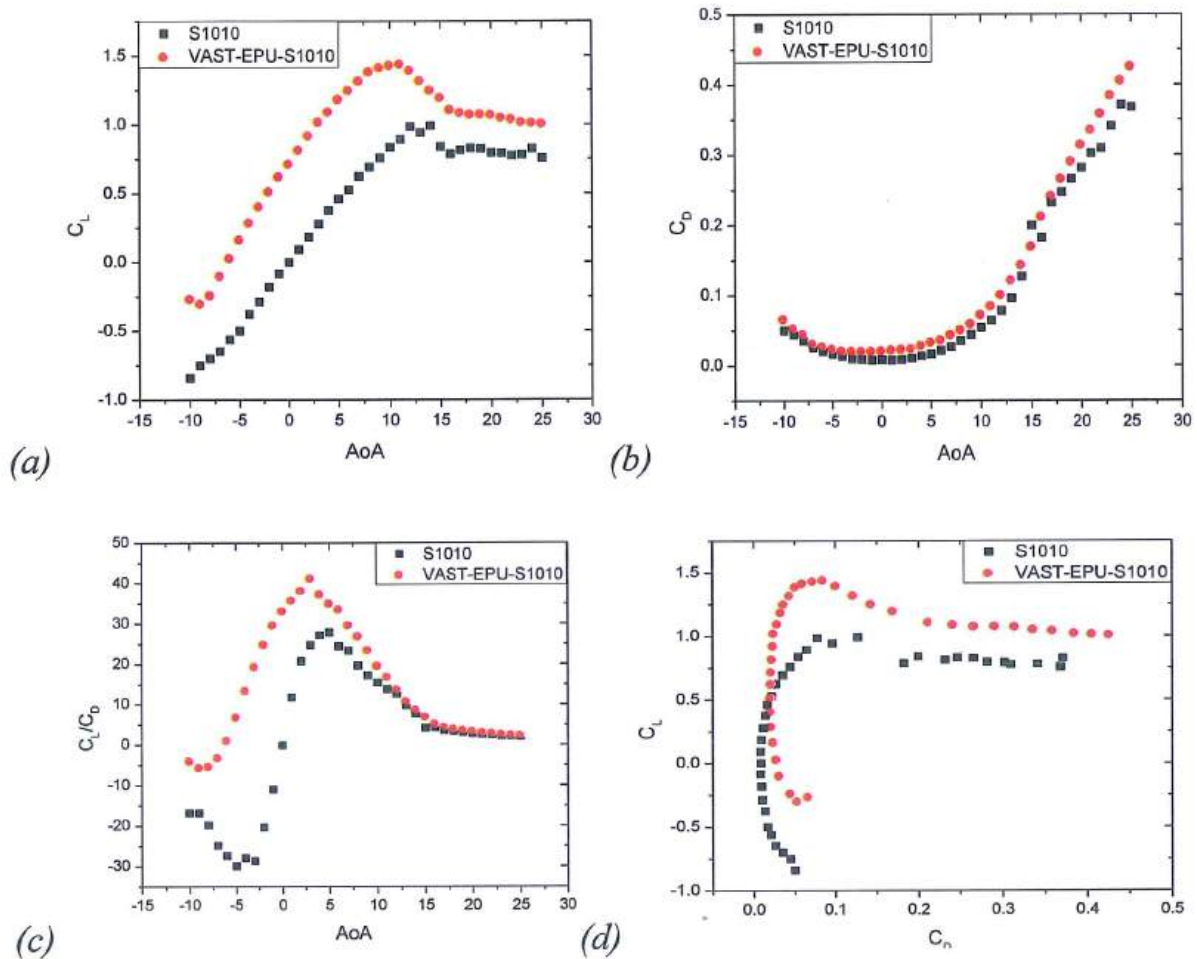
Hình 3.35. Các giá trị thu được của C_l (a), C_d (b), C_l/C_d (c), C_l so với C_d (d) của S1010 và VAST-EPU-S1010 khi hoạt động ở tốc độ gió 6,0 m/s
