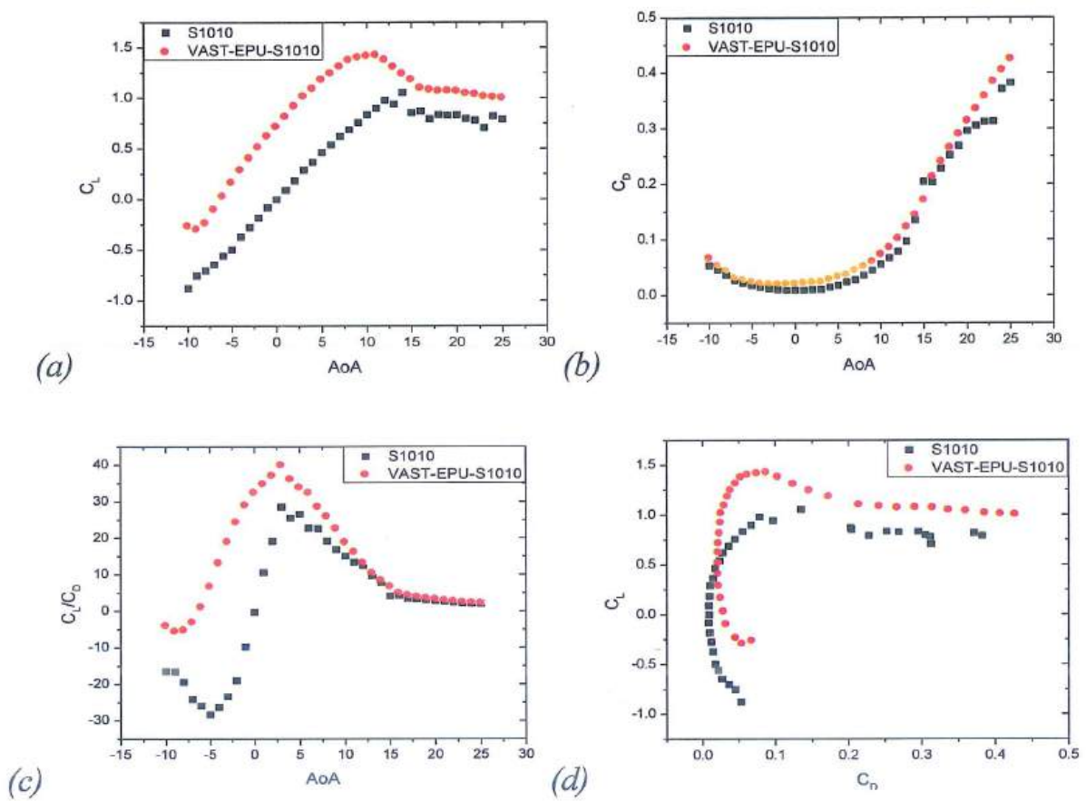
Hình 3.34. Các giá trị thu được của C_l (a), C_d (b), C_l/C_d (c), C_l so với C_d (d) của S1010 và VAST-EPU-S1010 khi hoạt động ở tốc độ gió 5,0 m/s
