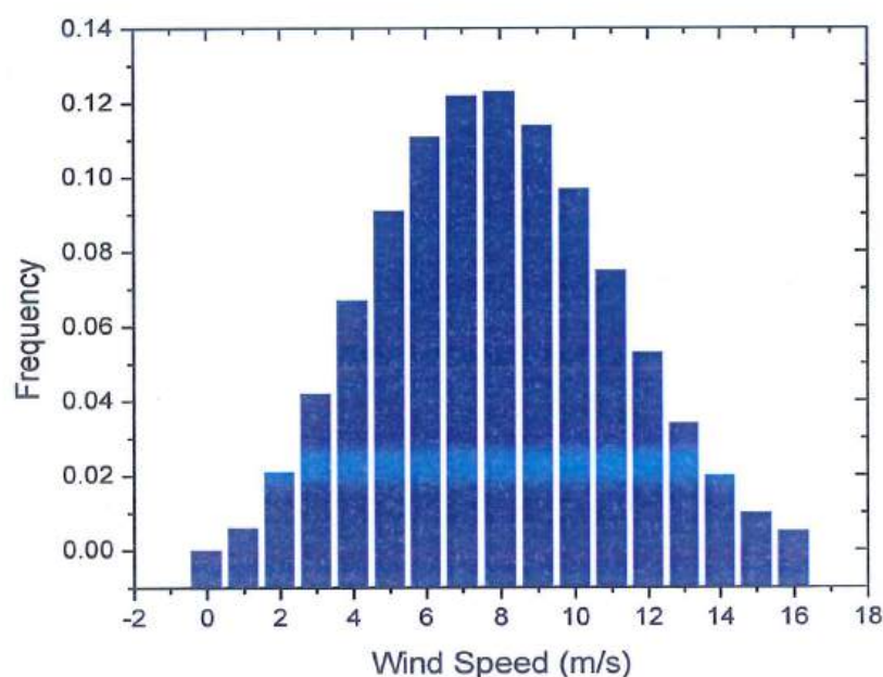
Hình 4.10. Hàm phân bố tốc độ gió Weibull trong khu vực trang trại
