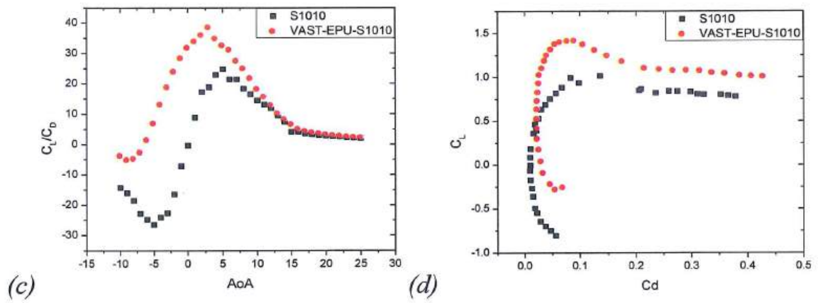
Hình 3.33. Các giá trị thu được của C_l (a), C_d (b), C_l/C_d (c), C_l so với C_d (d) của S1010 và VAST-EPU-S1010 khi hoạt động ở tốc độ gió 4,0 m/s
