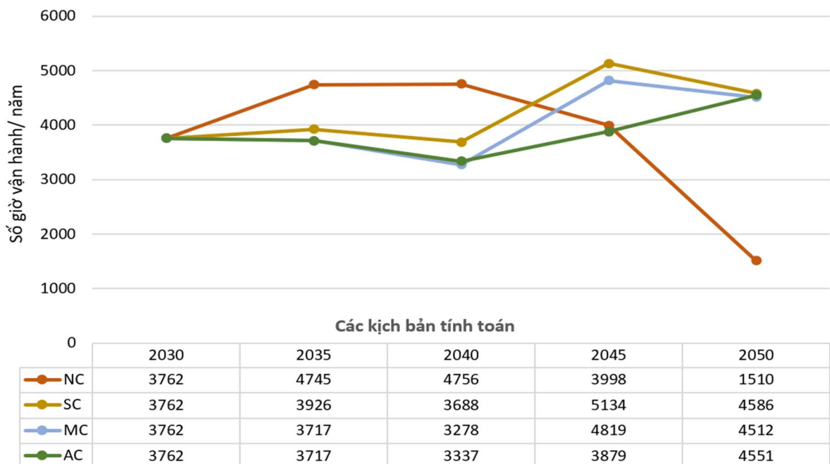
Hình 3.7 Kết quả tính toán số giờ huy động công suất phát của nhóm các NMD TBK theo các kịch bản
