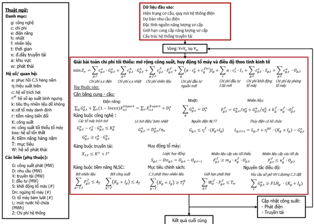
Hình 2.4 Cấu trúc thuật toán tính toán tối ưu của mô hình BALMOREL [35]
