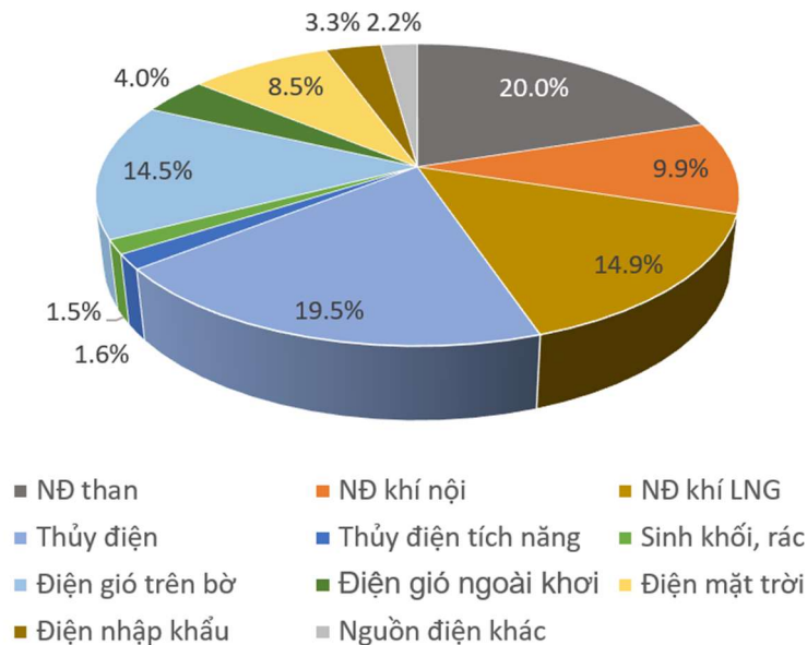
Hình 2.9 Cơ cấu nguồn điện toàn quốc năm 2030 [22]
