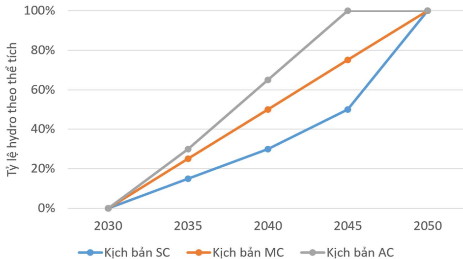
Hình 3.1a Các kịch bản nghiên cứu dựa trên tốc độ thâm nhập hydro khác nhau theo tỷ lệ thể tích phối trộn với KTN
