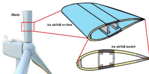
Hình 3.13. Minh họa thiết kế của cánh tuabin gió trục ngang.
