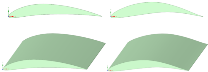
Hình 3.20. Biên dạng mẫu cánh NACA6409 và VAST-EPU-N6409
