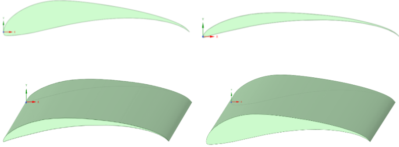
Hình 3.28. Biên dạng mẫu cánh S1223 và VAST-EPU-S1223
