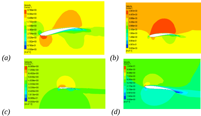
Hình 3.37. Đường đồng mức và xoáy khi tương tác với VAST-EPU-S1010: AoA = -5^\circ (a), AoA = 0^\circ (b), AoA = 5^\circ (c), AoA = 10^\circ (d) khi tốc độ gió 5,0 m/s
