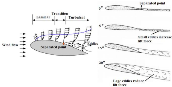
Hình 3.14. Minh họa các quá trình tương tác của gió với cánh
